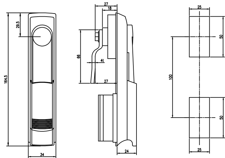
부착타공치수
